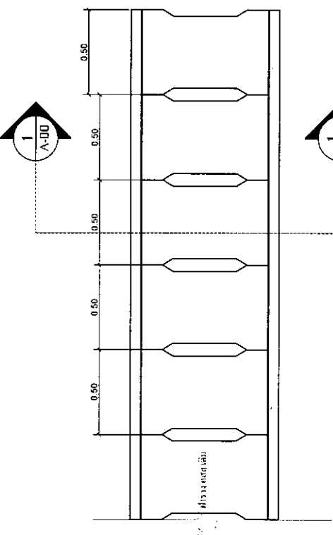
แปลนอาคารเรียน ขนาด ๐.๔๐ x ๐.๔๐ ม. มาตราส่วน 1:25
