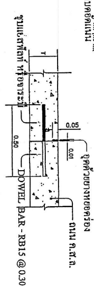
CONTRACTION JOINT 1 : 15 (ระยะ 10.00 ม.)
