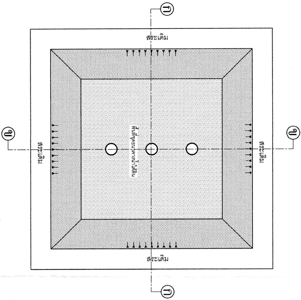
แบบแปลน NOT TO SCALE
