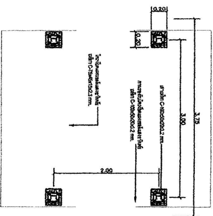
รูปที่ 3.1.2 เสาแบบ (ขนาดแบบแปลน 6 เมตร) 1:50
