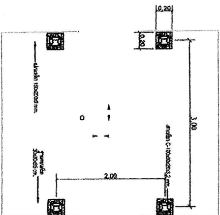
รูปที่ 3.1.1 เสาแบบ (ขนาดแบบแปลน 6 เมตร) 1:50
